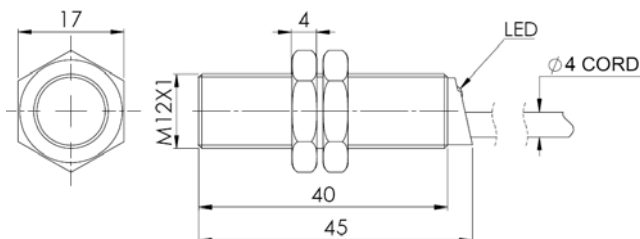
E2GN-M12KS02-WP-B1
