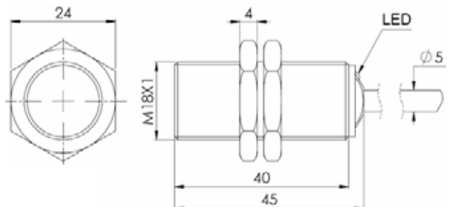
E2GN-M18KS05-WS-B1
